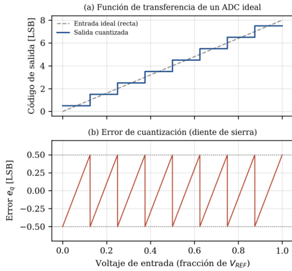
Figura 2. Función de transferencia de un ADC ideal (a) y error de cuantización asociado (b), para N_b = 3 bits.
