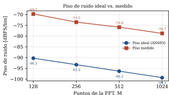
Figura 11. Piso de ruido ideal (AN693) frente al piso de ruido medido, para M = 128 a 1024 .
