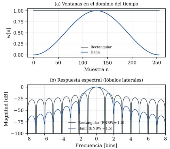
Figura 4. Comparación entre las ventanas rectangular y de Hann: (a) forma temporal; (b) respuesta espectral y lóbulos laterales.
